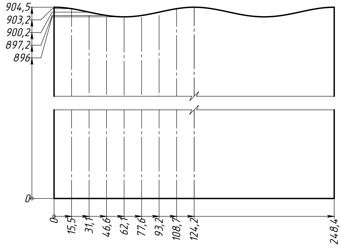
Поз.2 (Труба) развертка 1 : 2
