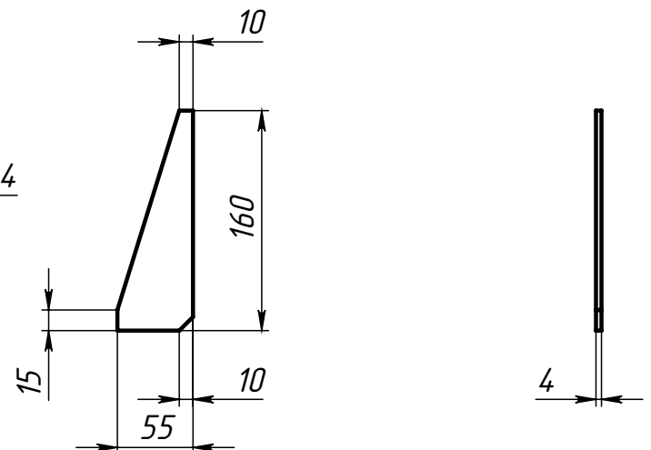
Поз.4 (Косынка)
