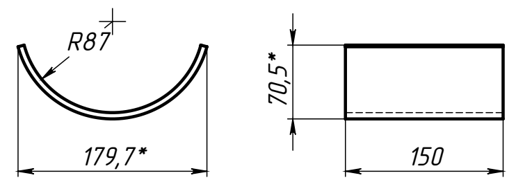
Поз.3 (Накладка)
